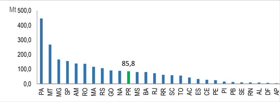
GRÁFICO 15 - EMISSÃO DE CO 2 NO BRASIL E NOS ESTADOS - 2021
